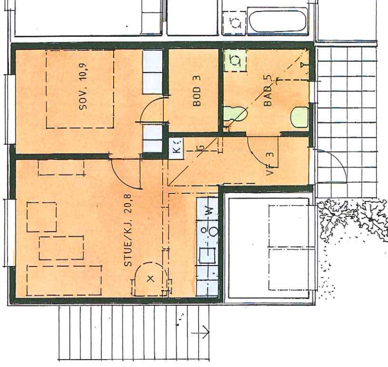
PLAN 1. ETASJE
